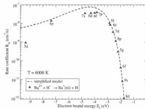
Рис. 4: Константы скоростей K_f(T) процессов взаимной нейтрализации, происходящих при столкновениях Ba^{2+} + H^- , для температуры T = 6000 К как функция энергии связи конечного состояния f . Треугольниками обозначены результаты многоканальных расчетов, пунктирной линией показаны результаты применения упрощенного модельного подхода.
