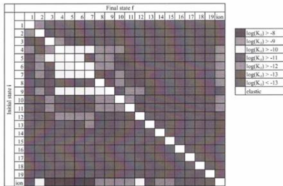
Рис. 3: Графическое представление констант скоростей (в см 3 /с) для столкновений ионов бария и водорода при температуре T = 6'000 К.
