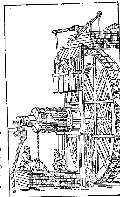
Водяной двигатель.
